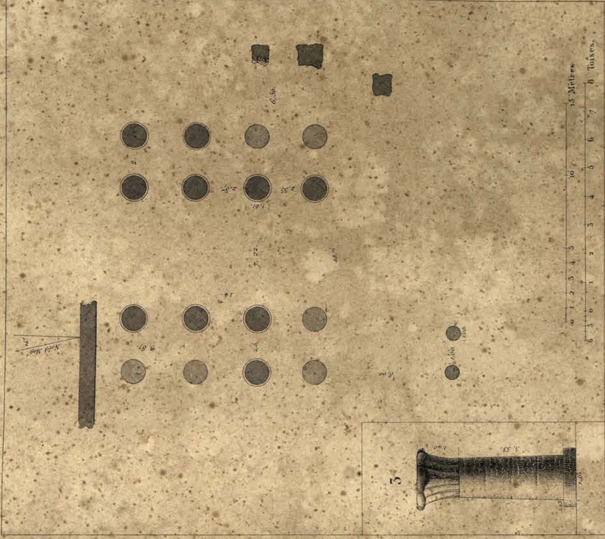
1. PLAN GÉNÉRAL DES RUINES. 2. 3. PLAN DES RESTES D'UN ANCIEN ÉDIFIKE ET ÉLEVATION D'UNE COLONNE.
