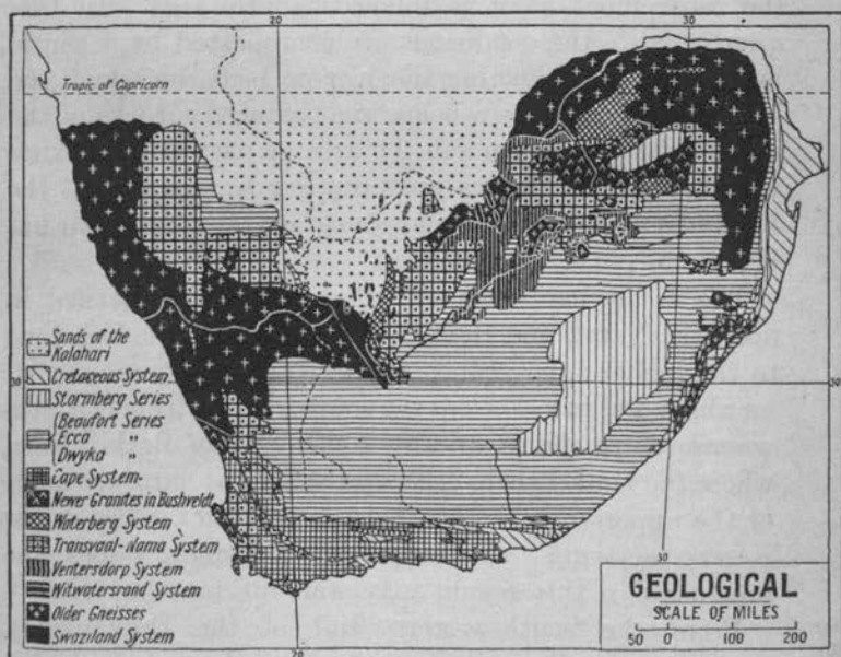
FIG. 8. Geology.
